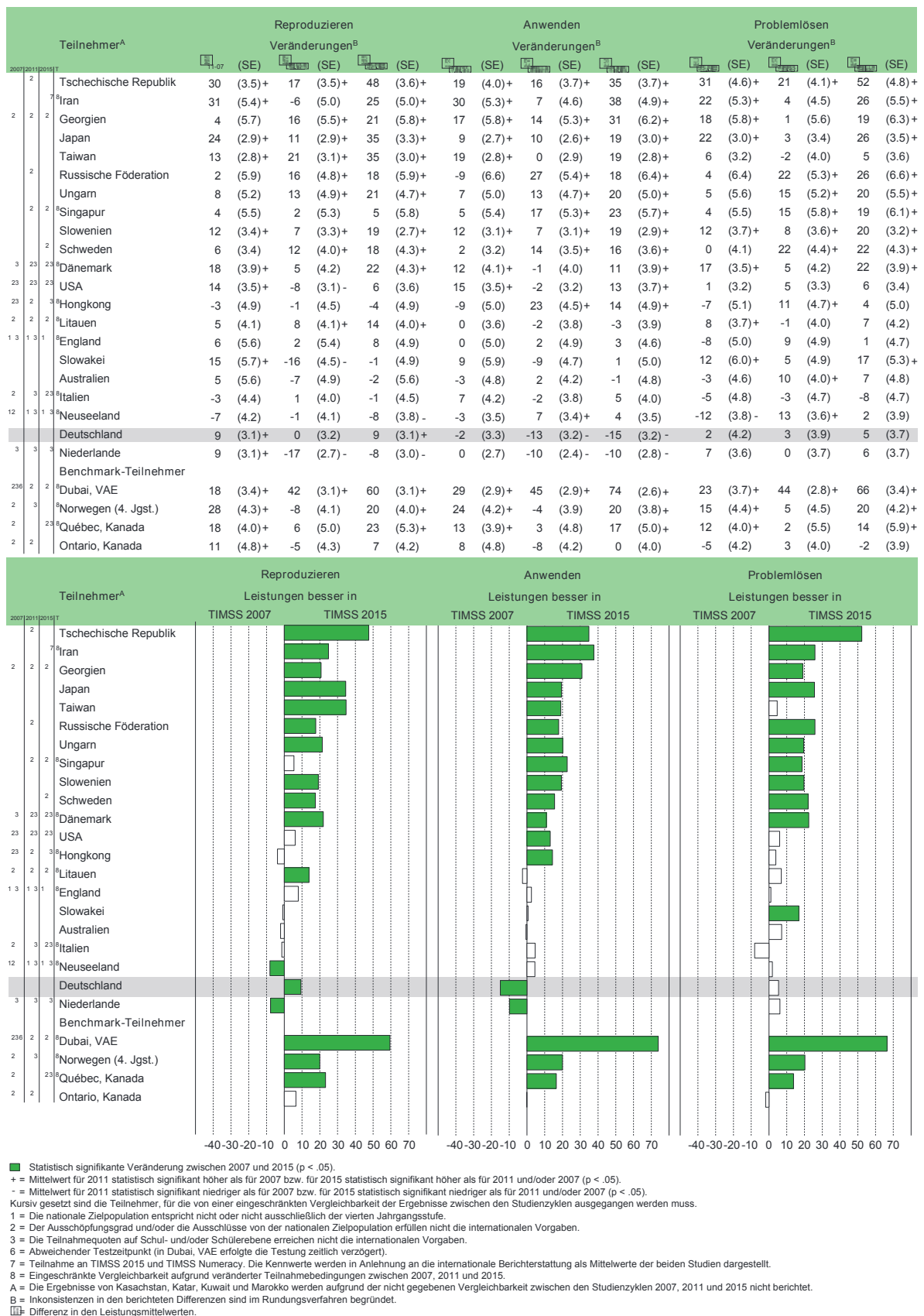
Abbildung 3.13: Vergleich der Testleistungen in Mathematik zwischen TIMSS 2007, 2011 und 2015 in den kognitiven Anforderungsbereichen Reproduzieren, Anwenden und Problemlösen II
